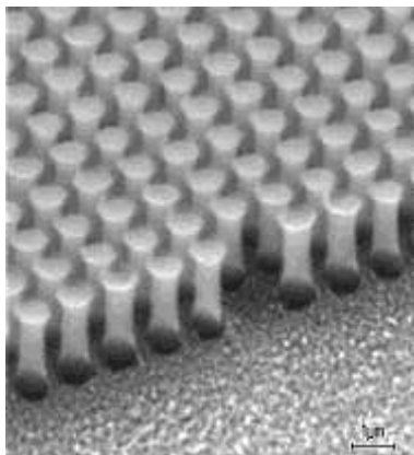
Рис.32. «Липучка»: а) структура, выращенная с помощью плазменной технологии и перенесенная на гибкую основу, б) ладонь игрушки, на которую нанесен этот «материал» выдерживает вес в 400\text{г/см}^2
