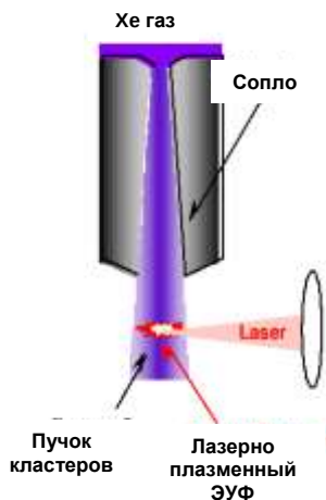
Рис.33 Лазерно-плазменный источник ЭУФ на кластерах ксенона
