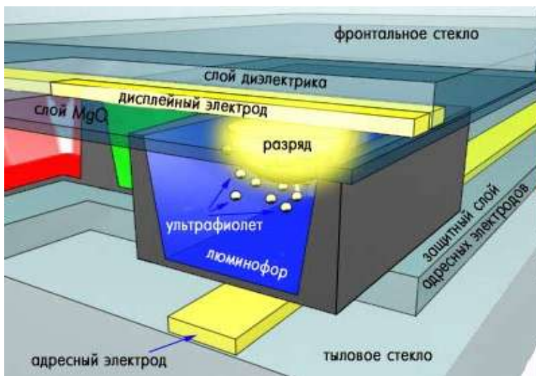
Рис.24. Устройство ячейки плазменного дисплея
