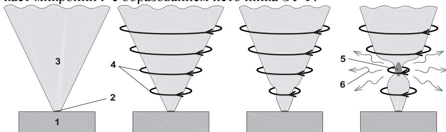
Рис.34. Возникновение ЭУФ при инициированном лазером микропинче: 1 – катод, 2 – катодный факел, 3 – плазма, 4 – магнитное поле, 5 – микропинч, 6 – ЭУФ излучение
