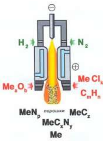
Рис.27. Плазменно-струйный метод получения нанопорошков
