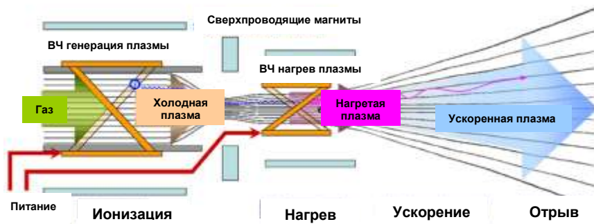
Рис.46. Схема работы плазменного двигателя VASIMR
