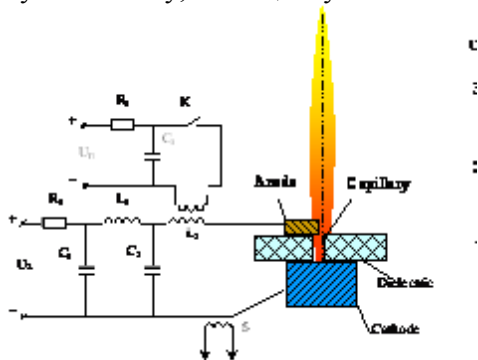
Рис.36. Факельный разряд и его электрическая схема
