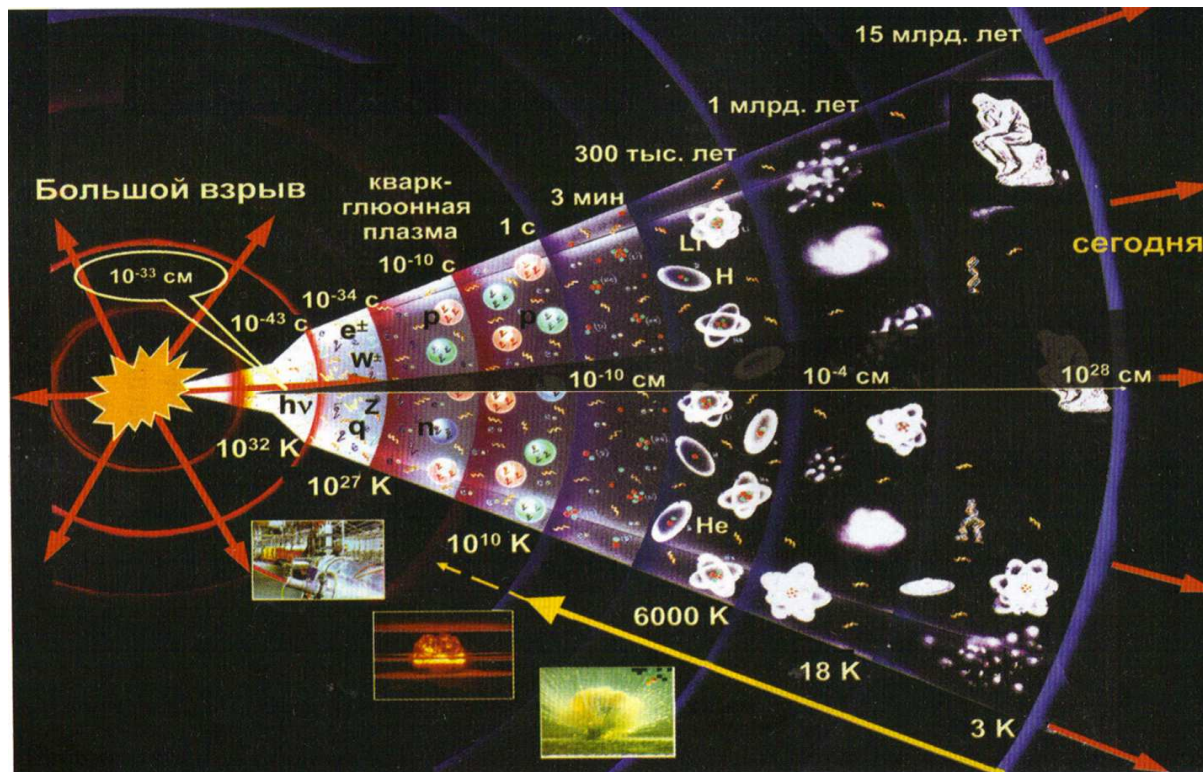
Рис.1 Эволюция Вселенной согласно теории Большого Взрыва (по [1])
