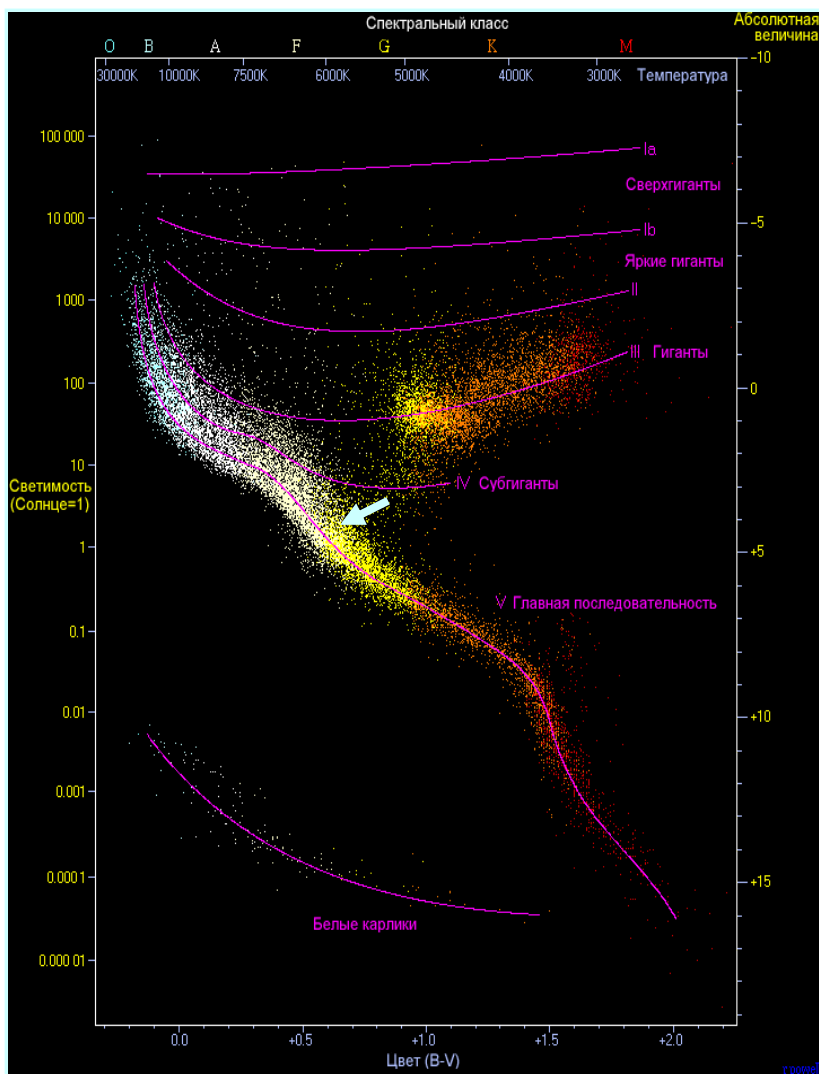
Рис. 6. Классификация наблюдаемых звезд. Стрелочкой указано место нашего Солнца
