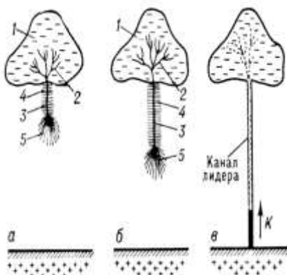
Рис.18. Схема развития наземной молнии: 1 – облако, 2 – стримеры. 3 – канал ступенчатого лидера. 4 – корона канала, 5 – импульсная корона на головке канала.
