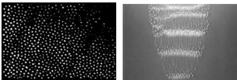
Рис.40. Плазменные кристаллы: а) кристалл из сфер MgO размером в 2-3 мкм, б) волны в плазменном кристалле.
