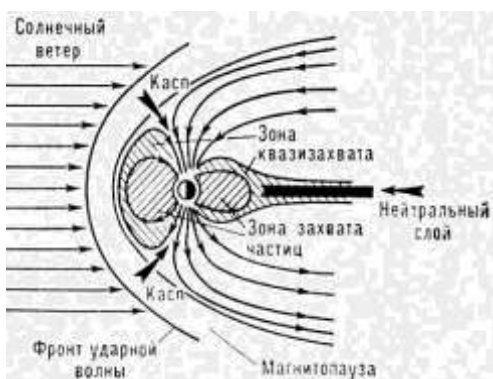
Рис.14а. Схема взаимодействия солнечного ветра с магнитным полем Земли с учетом его неоднородной структуры с дневной и ночной сторон
