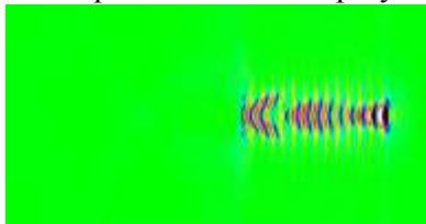
Рис. 37. Моделирование поля и плазмы в коротком лазерном импульсе
