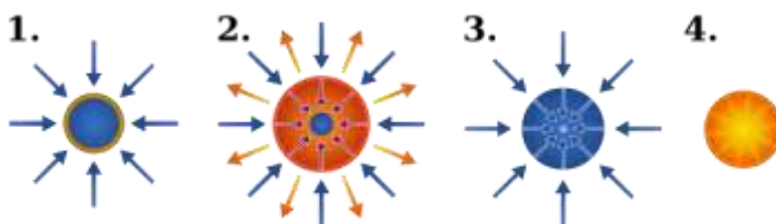
Рис.42. Процессы при ИТС: 1- образование плазменной короны под действием лазерного излучения, 2 - реактивное действие потоков газа сжимает шарик, 70% вещества испаряется, остальное сжимается в 10 000 раз, 3 - ударная волна нагревает центр до 10 кэВ, 4 - термоядерное горение
