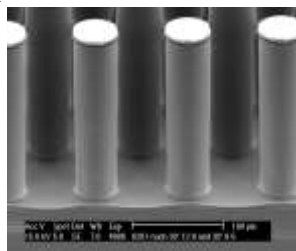
Рис.30. Столбчатая структура, полученная плазменным травлением
