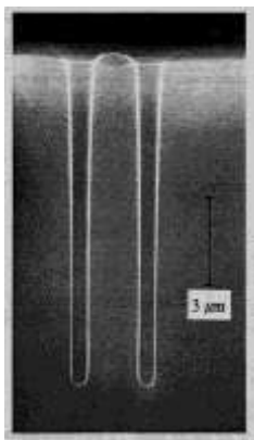
Рис.29. «Тренчи» в Si, полученные плазменным травлением
