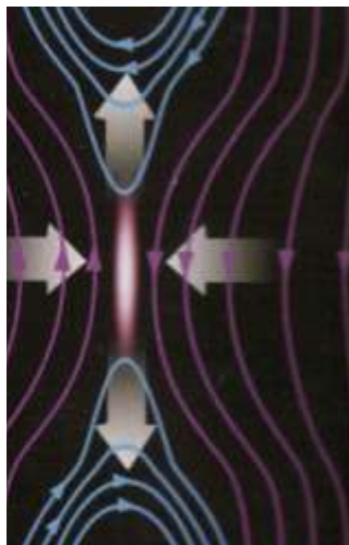
Рис.11. Перезамыкание магнитных силовых линий
