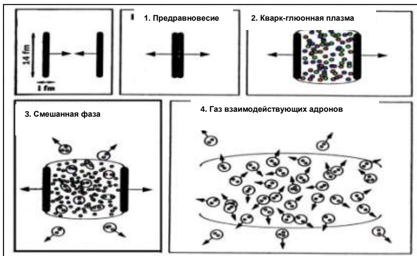
Рис.38. Процессы при центральном столкновении релятивистских ядер золота (из доклада В.М.Емельянова, В.А.Огорокова и М.Н.Стриханова на зимней научной сессии МИФИ в 2006 году)
