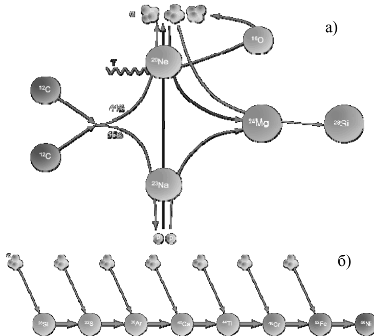
Рис.5а,б. Синтез более тяжелых элементов
