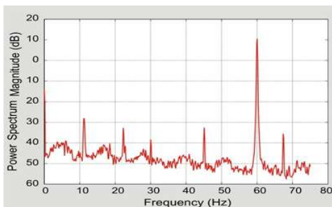
Рис.17. Спектр частот резонатора Шумана.
