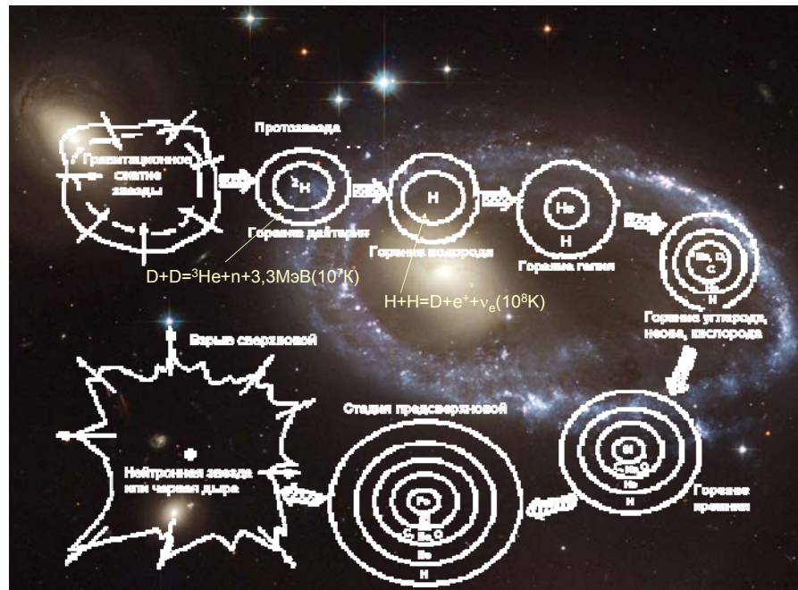
Рис.3. Эволюция звезд при термоядерном горении.
