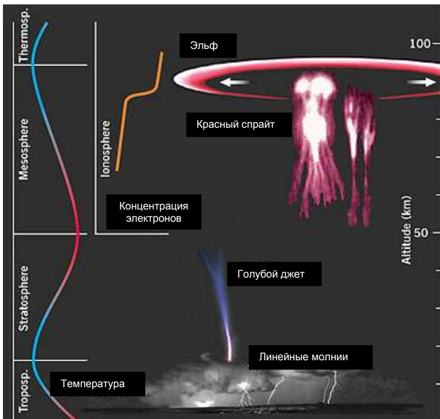
Рис.21. Новые плазменные эффекты недавно обнаруженные в верхних слоях атмосферы
