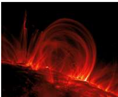
Рис. 10. «Фонтаны огня»
