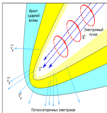
Рис.19. Процессы во фронте лидера молнии
