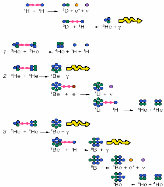
Рис.4 Протонный цикл ядерных превращений
