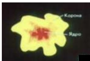
Рис.43. Неустойчивость Релея-Тейлора
